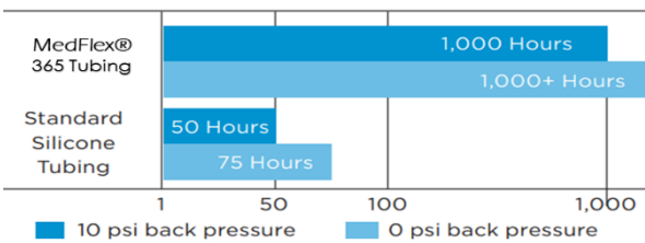
左图 (室温、水介质、零背压) 条件下: 尺寸为 6.4mm*9.5mm 的软管在 600RPM 的三轮蠕动泵驱动下连续不间断工作时长达 1000hrs。
